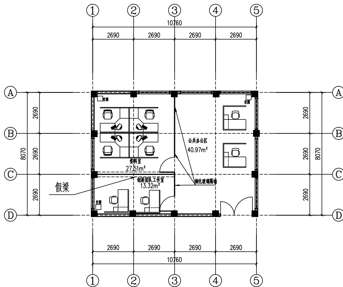
电力实训楼资料室平面图
