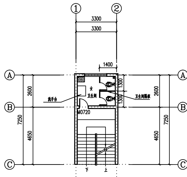
信息楼卫生间平面图 第二、四层女卫生间
