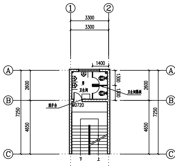
信息楼卫生间平面图 第三、五层男卫生间
