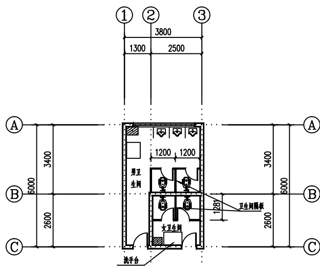
电力实训楼卫生间平面图 第一、二、三、五层
